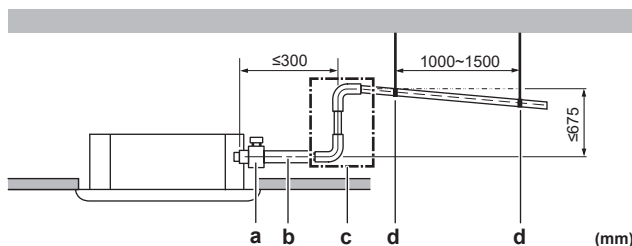
a Metallschelle (Zubehör) b Ablaufschlauch (Zubehör) c Abflussrohr ansteigend (Vinylrohr mit 25 mm Nenndurchmesser und 32 mm Außendurchmesser) (bauseitig zu liefern) d Aufhängungen (bauseitig zu liefern)
