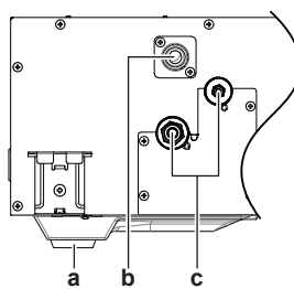
a Abfluss-Auslass für Wartungsarbeiten b Abflussrohr-Anschluss c Kältemittelleitungen
