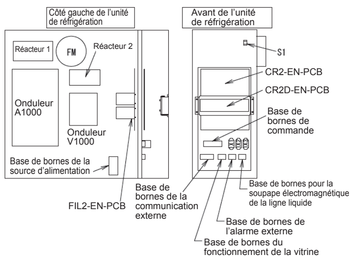
Disposition interne du boîtier électrique
