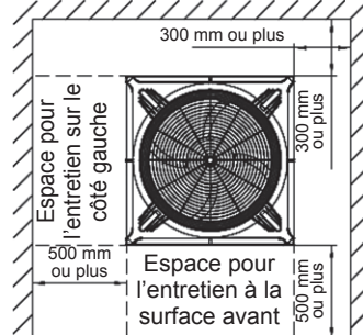
En présence d'un mur sur trois côtés
