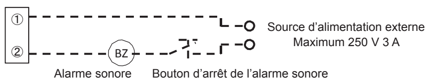
Base de bornes de l'alarme externe
