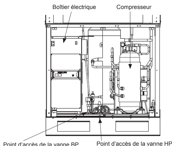
Façade avant de l'unité de réfrigération
