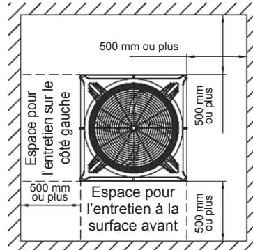
En présence d'un mur sur les quatre côtés
