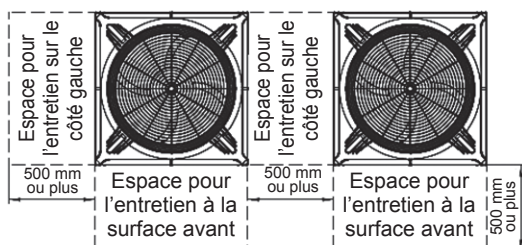
Installation en série
