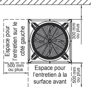
En présence d'un mur sur un côté
