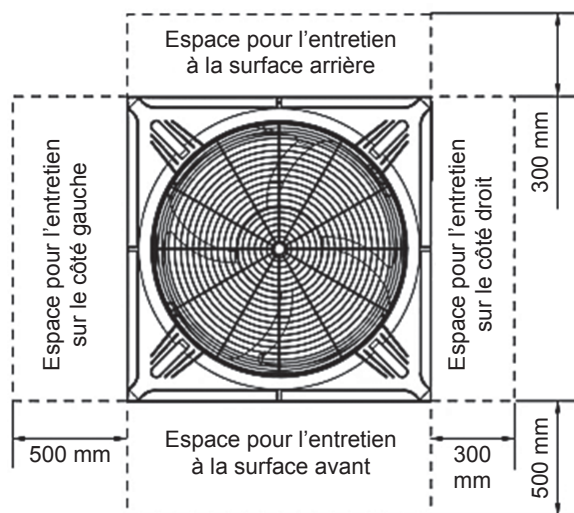
En présence d'un mur sur un côté
