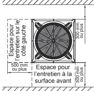
En présence d'un mur sur deux côtés
