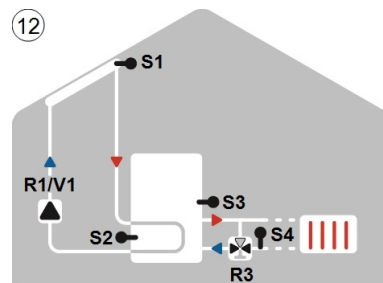
12 Solar mit Rücklaufanhebung
