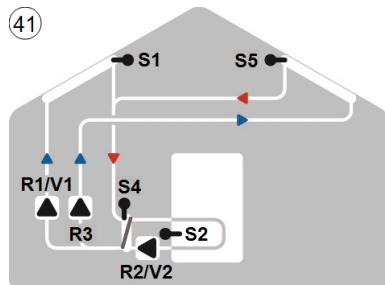
41 Solar mit 2 Kollektoren, Wärmetauscher und 3 Pumpen
