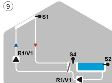
9 Solar mit Wärmetauscher und Pool
