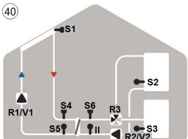
40 Solar mit Wärmetauscher, 2 Speicher und Ventil
