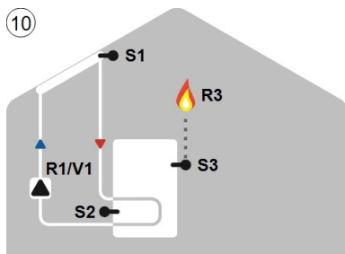
10 Solar mit Thermostat
