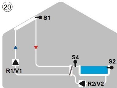
Solar mit Pool und Wärmetauscher
