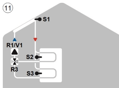
11 Solar mit 2 Zonenspeicher
