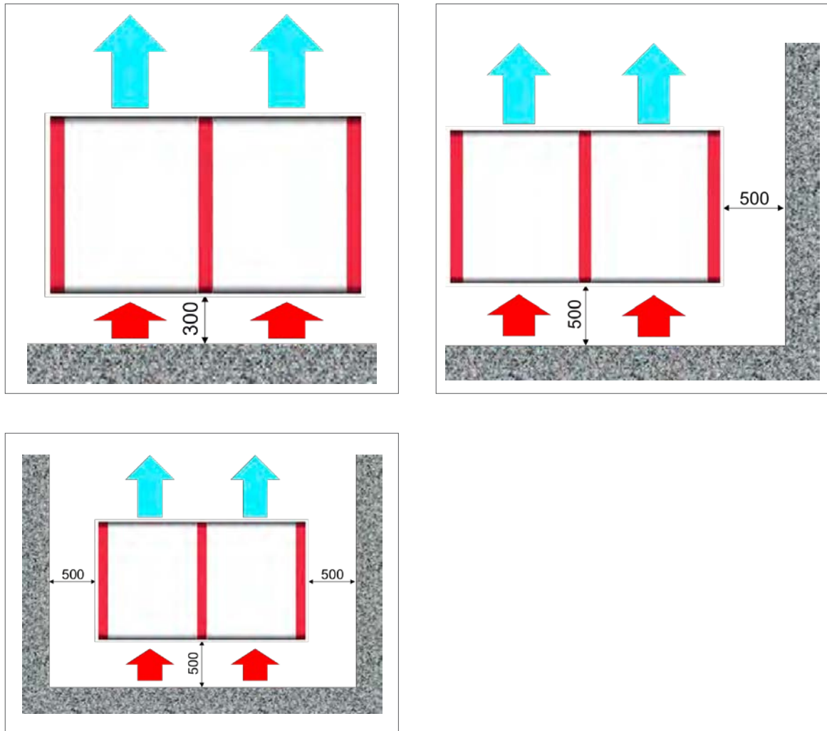
Fig. 8: Ulteriori varianti di installazioni; esempio per HPS240
