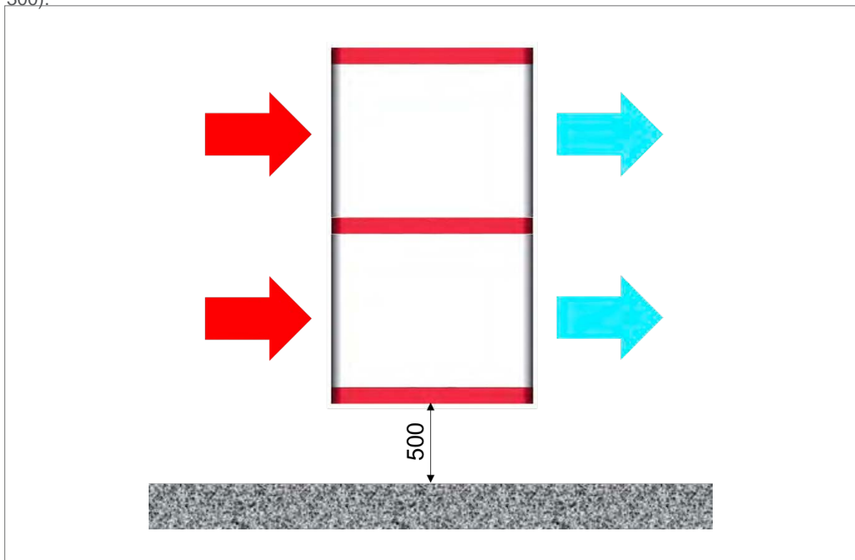
Fig. 7: Variante di installazione raccomandata dal produttore; esempio per HPS240
