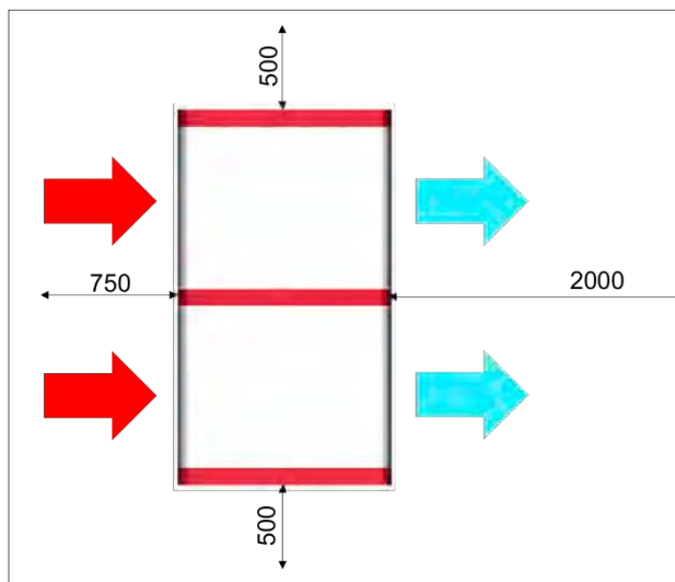
Fig. 4: Distanze minime consigliate: esempio per il Silent Source 240
