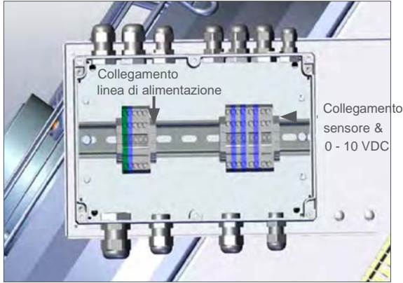
Fig. 9: Scatole di giunzione con morsettiere sull'evaporatore esterno Silent Source HPS240 e HPS300 (2 x)
