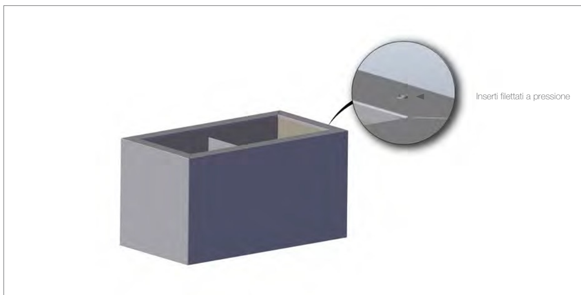
Fig. 6: Basamento in alluminio (sx) e inserti filettati a pressione (dx); esempio per HPS240
