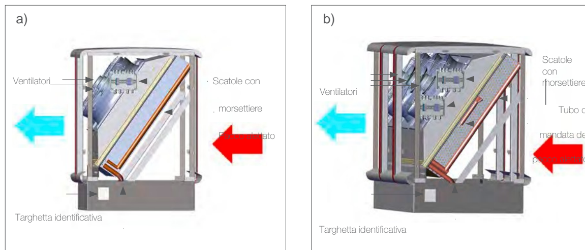
Fig. 3: Componenti dell'evaporatore esterno; a) Silent Source 240, b) Silent Source 300
