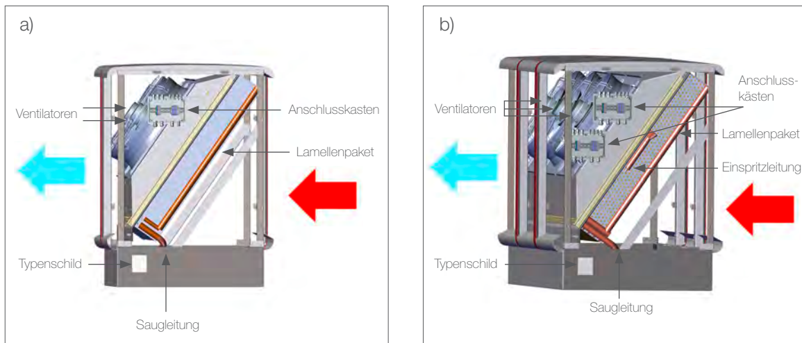
Abb. 3: Komponenten des Außenluftverdampfers; a) Silent Source 240, b) Silent Source 300
