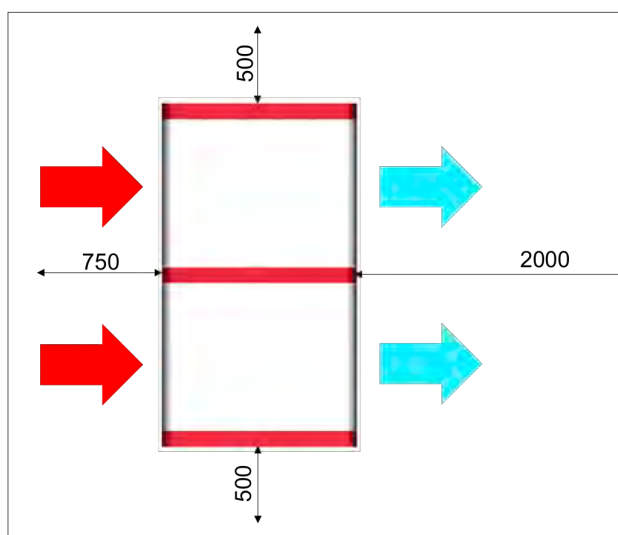
Abb. 4: Empfohlene Mindestabstände, hier exemplarisch für Silent Source 240
