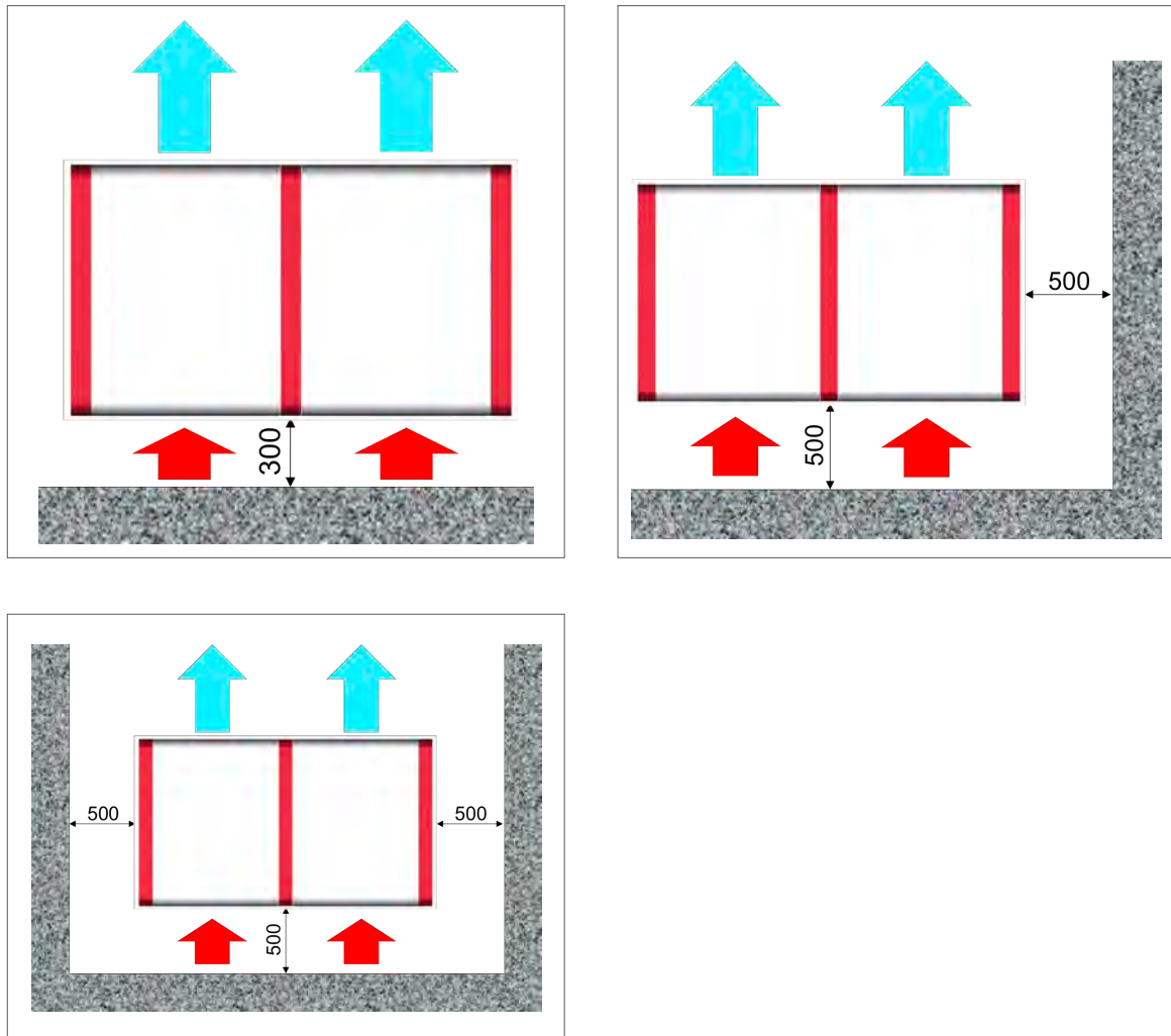
Abb. 8: Weitere mögliche Aufstellungsvarianten; hier exemplarisch für HPS240
