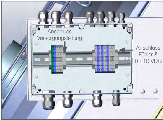
Abb. 9: Elektrische Anschlusskästen am Außenluftverdampfer Silent Source HPS240 und HPS300 (2 x)
