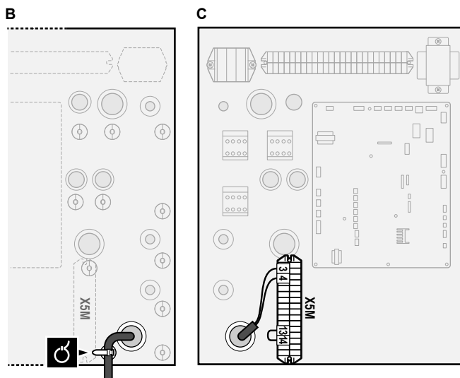
S4S Smart Grid-Impulszähler
